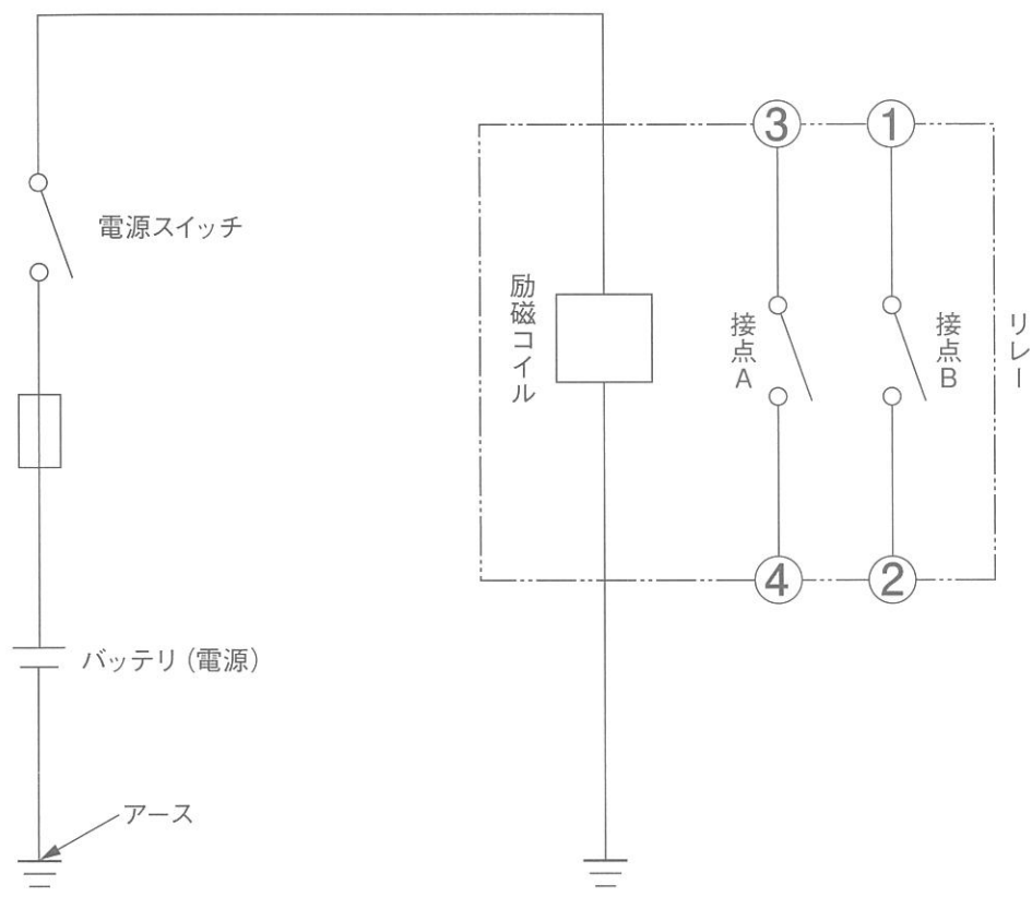
〈リレーの回路図〉
